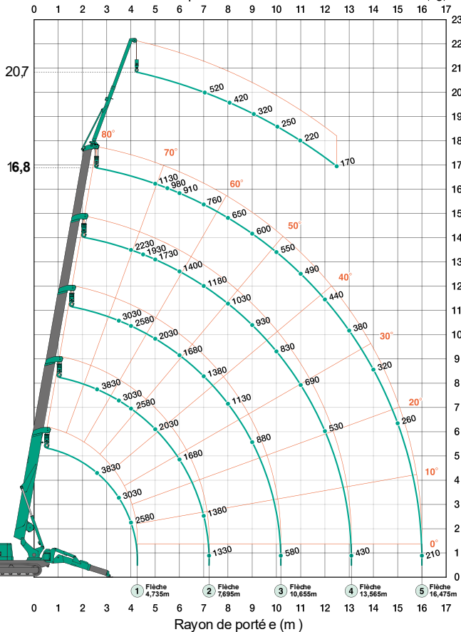
MC405 Stabilisateurs en position maximum (kg)
