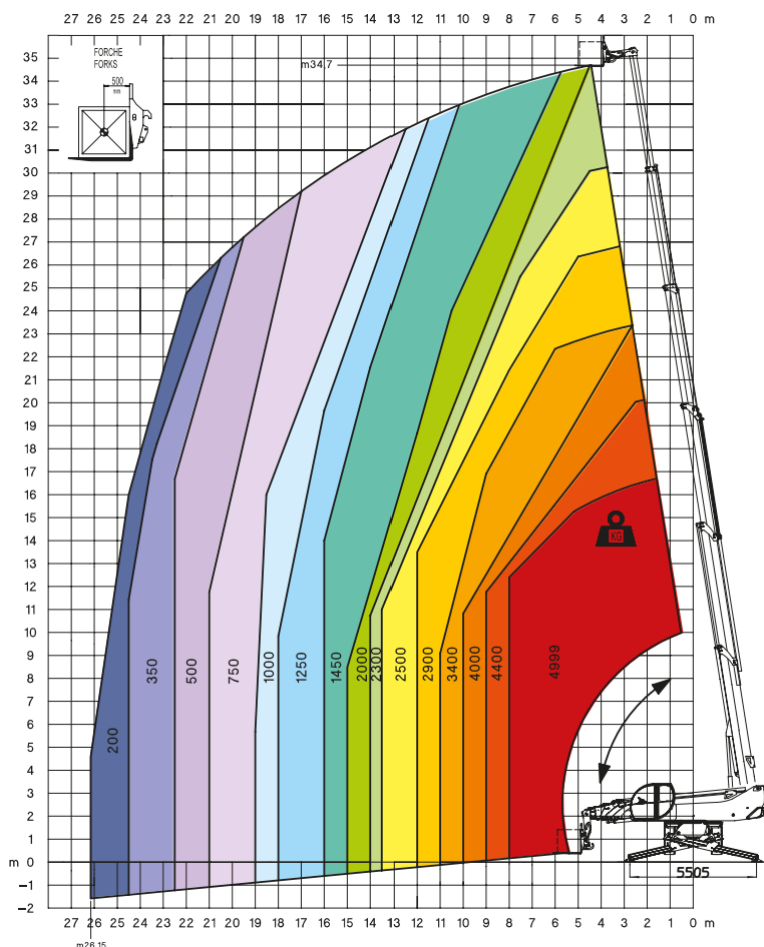
Abaque de charge sur stabilisateurs déployés en rotation avec fourches
